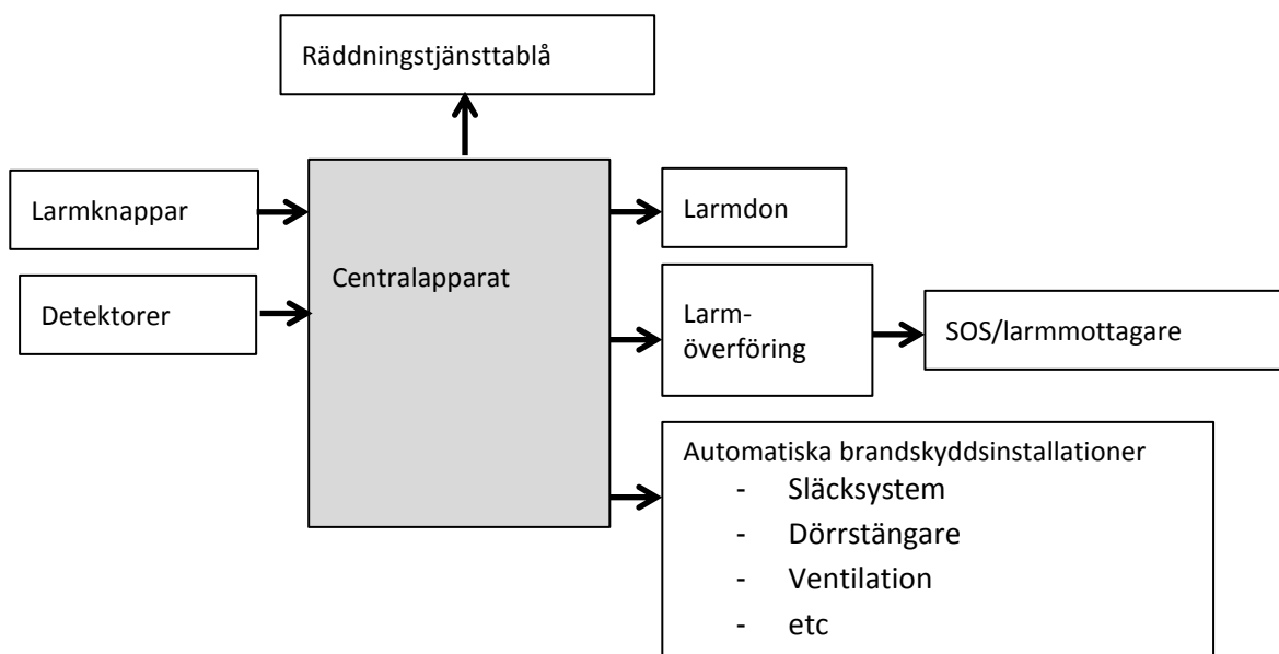
Figur 16: Komponenter i ett automatiskt brandlarm.
