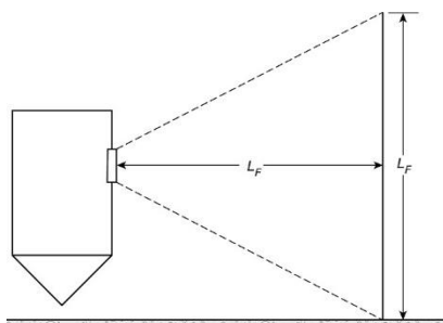
Figur 6: Illustration av dimensioner på eldklot (från NFPA 68)
