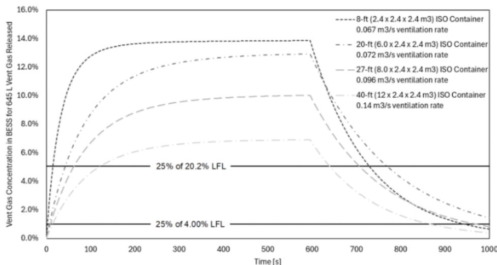
Figur 9: Ventilationsgaskoncentrationer över tid för 154 l gas frigjord per cell för 8-cells TR-händelse i olika BESS ISO-behållare med 20 % antagen fri luftvolym för NFPA 69 minsta erforderliga ventilationshastighet och 10,8 l/s gasutsläppshastighet (ungefär 1 cell/minut TR-utbredningshastighet). [62]
