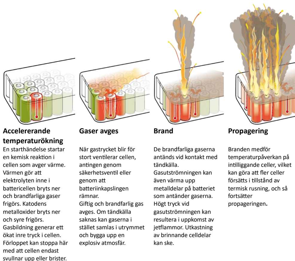
Figur 3. Schematisk översikt över brandförlopp i litiumjonbatteri, illustration Fredrik Saarkoppel/ Brandskyddslaget AB.
