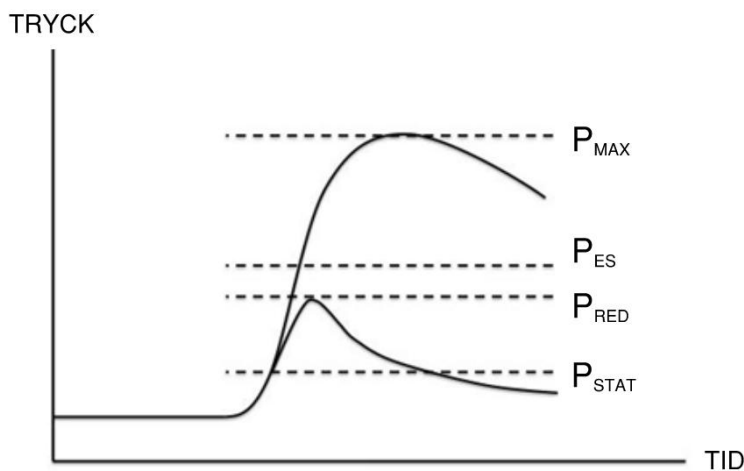
Figur 5: Tryckförhållandet i en behållare/container under ett explosionsförlopp
