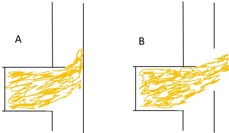
Figur 7 De varma gaserna leds mot den yttre glastrutan så att den går sönder och ventilerar rökgaserna [12].
