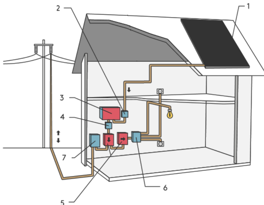
Figur 10. Huvudkomponenterna i ett solcellssystem, 1 = solceller, 2 = DC-brytare, 3 = växelriktare, 4 = AC-brytare, 5 = elmätare, 6 = husets elcentral och 7 = extern nätslutning. Anpassad från [Kovács, 2018].
