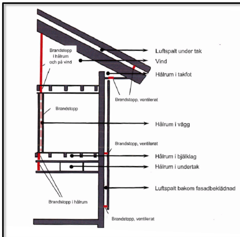
Figur 3: Olika brandspridningsvägar i hållrum. De röda markeringarna visar var brandstopp bör vara installerat. Bild hämtad från Brandsäkra trähus, version 3 [16].
