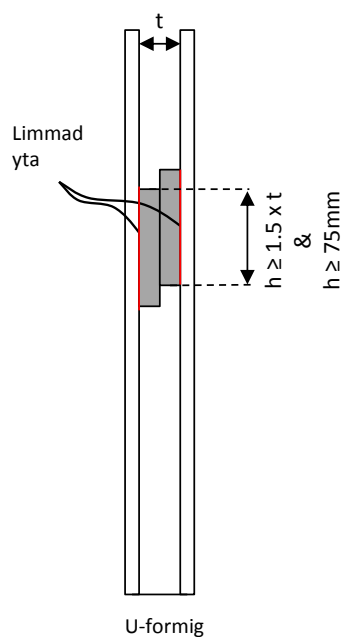
Figur 18. Schematisk installation av brandstopp (röda pilar visar möjliga rörelser hos delar av byggnadselementet). Installationshjälp visas t h.
