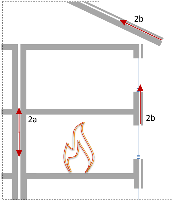
Figur 13. Potentiella brandspridningsvägar genom hålrum.
